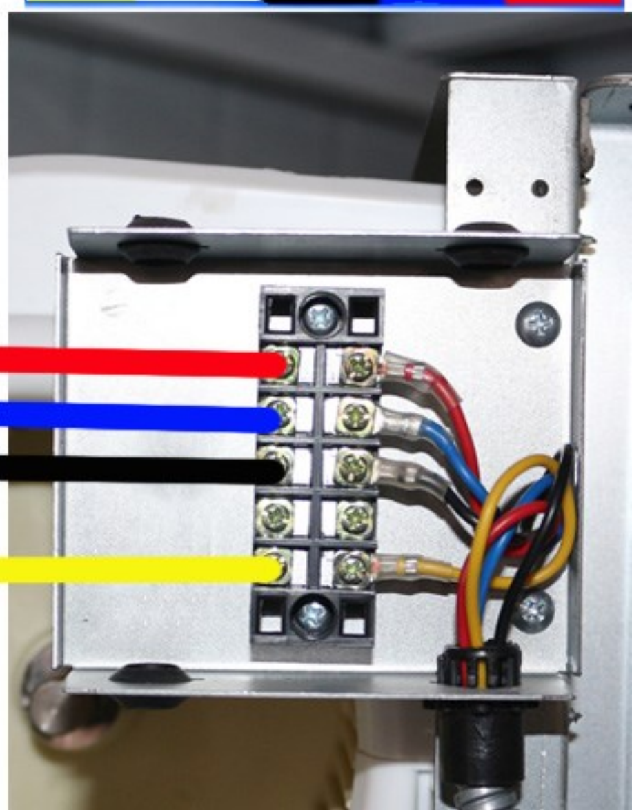
风机盘管接线盒端口
