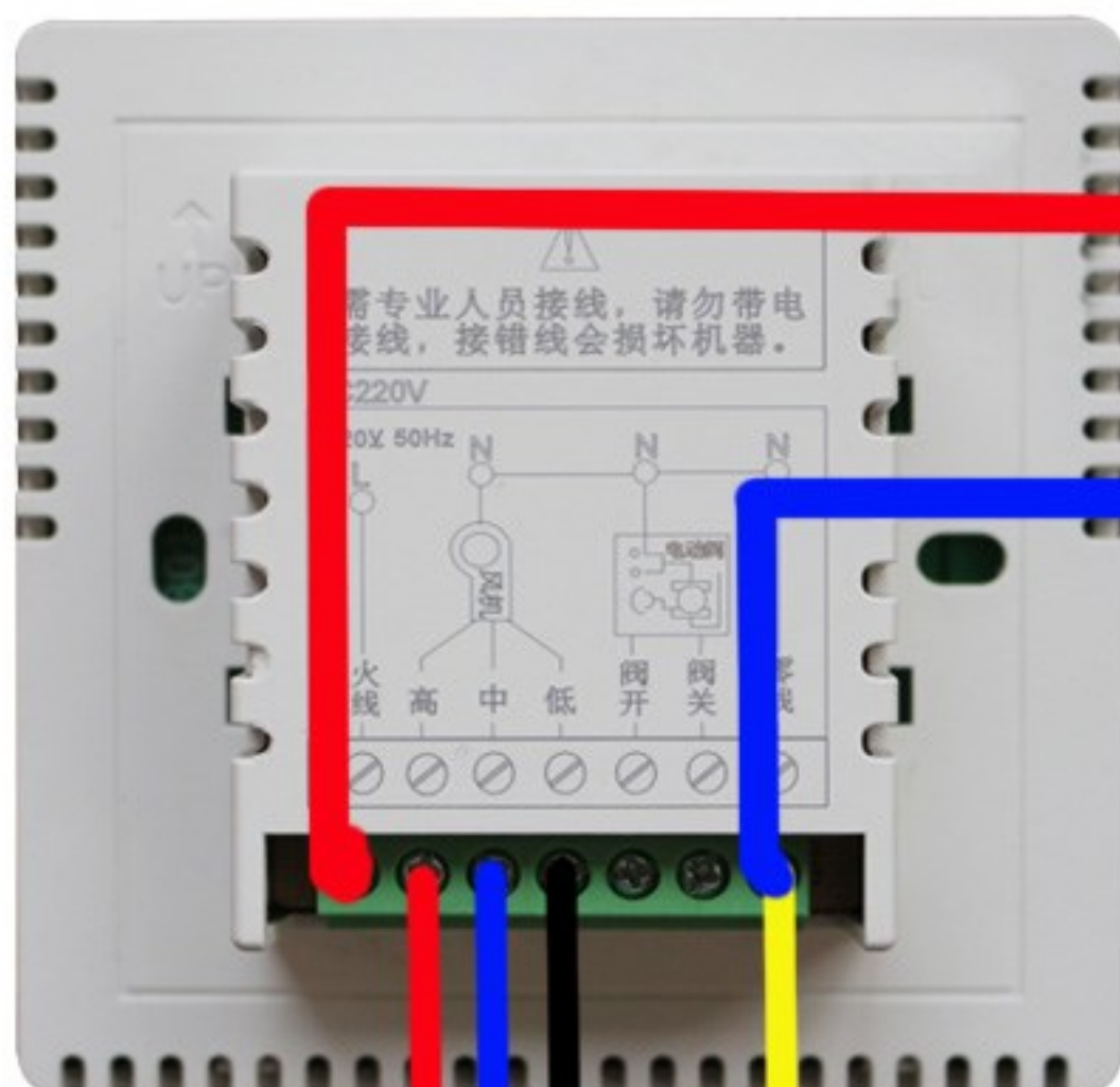
中央空调液晶温控器
