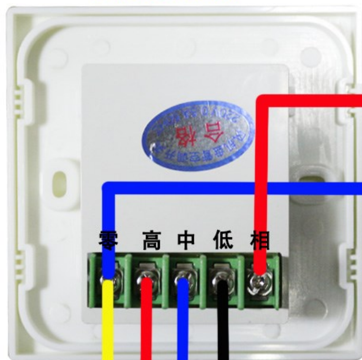
三速开关控制器
